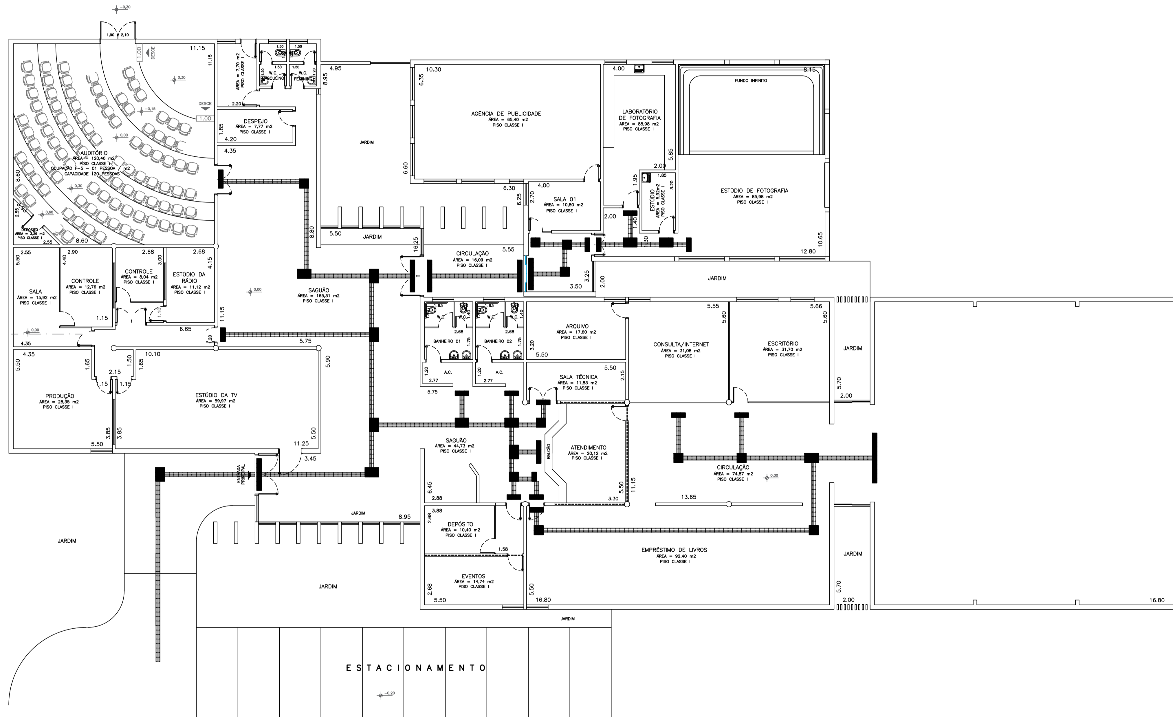
PLANTA BAIXA DA BIBLIOTECA E DA AGÊNCIA DE PROPAGANDA Escala - 1:100
